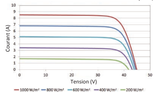
Courant - Tension courbe à différents niveaux de luminosité (156M/72)
