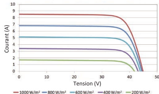
Courant - Tension courbe à différents niveaux de luminosité (156M/72)
